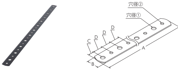
フリープレート チドリ 15X300
