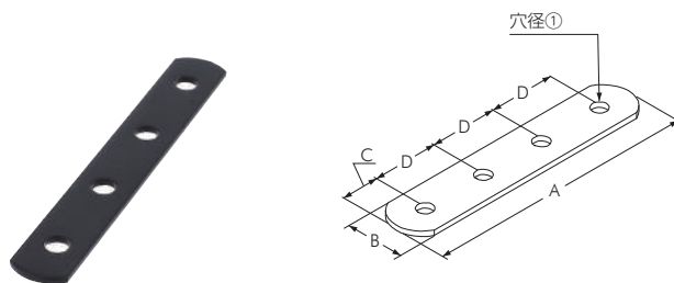
ジョイントプレート A-8
