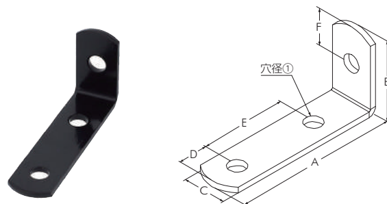
ジョイントプレート D-2
