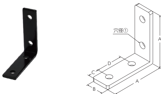
ミニジョイント アングル K-2
