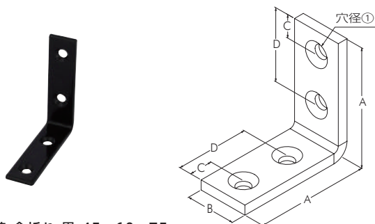
塩ビ塗装 金折れ 黒 45・60・75mm
