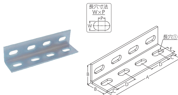
ユニクロ ファンブル 120・150mm
