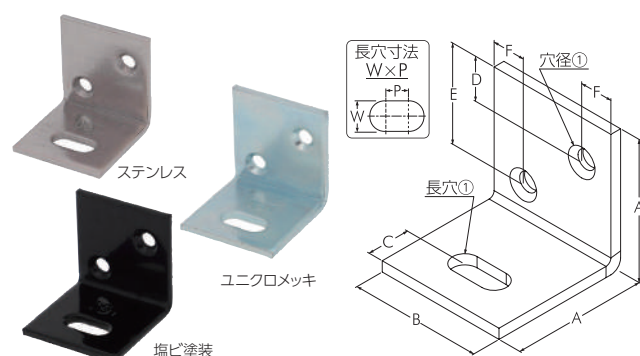
金折れ鋼板 横穴
