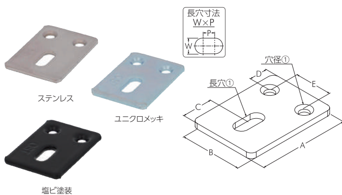
平鋼板 縦穴
