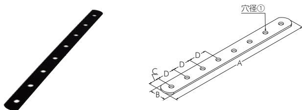
ジョイントプレート A-7
