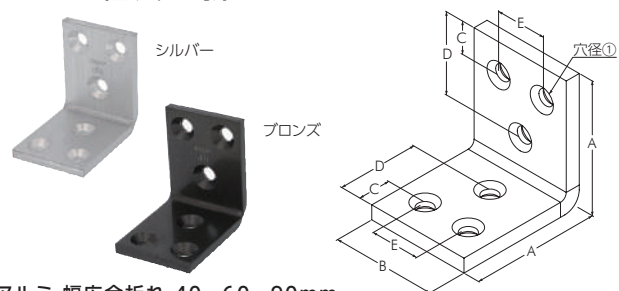
アルミ 幅広金折れ 40・60・90mm
