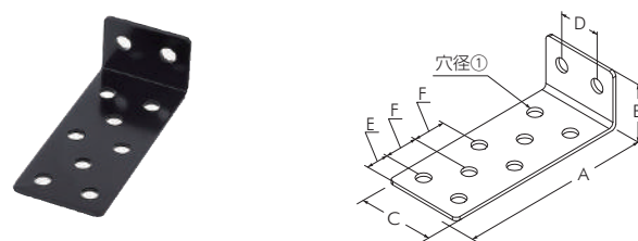
ミニジョイント 金折れ N-4
