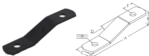
ジョイントプレート D-1
