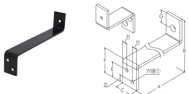
ジョイントプレート H-2
