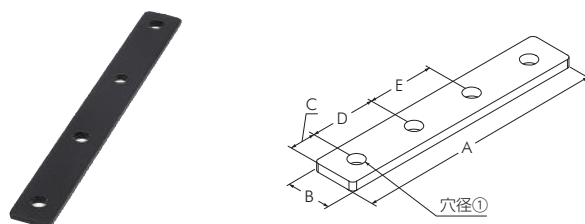
ミニジョイント プレート K-9
