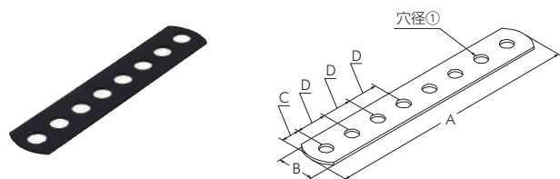
フリープレート ストレート 20X100
