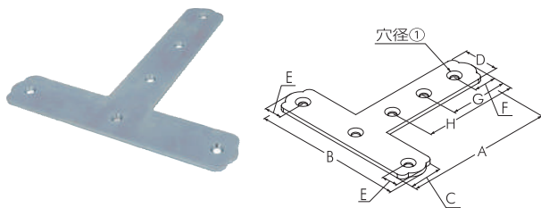
ユニクロ T字 150・180mm
