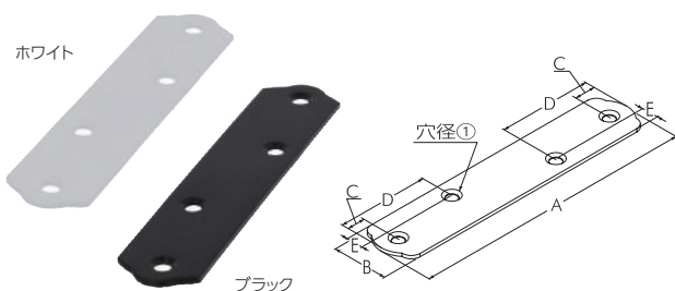
カラープレート 小・中
