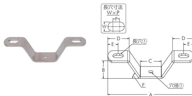
ジョイントプレート E-1
