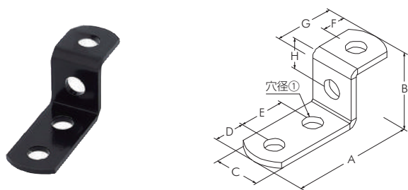
ジョイントプレート F-2
