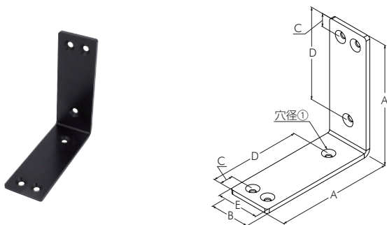
L 字金具
