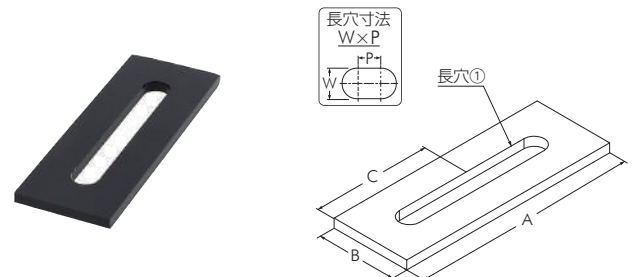
ジョイントプレート G-3
