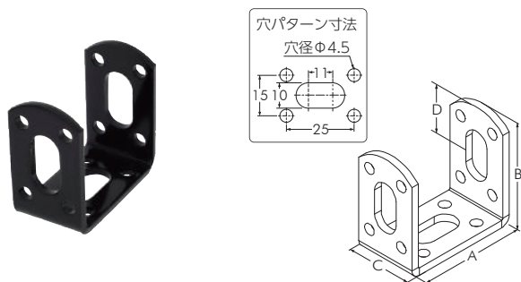
ジョイントプレート C-1
