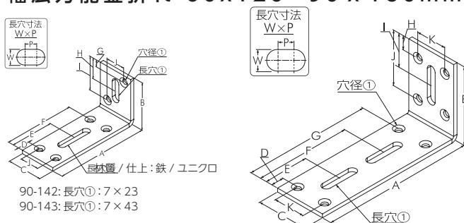
幅広万能金折れ 60x120・90x180mm
