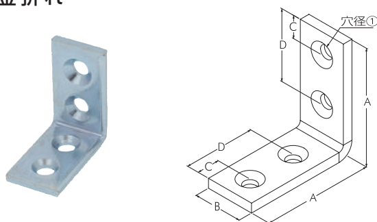
特厚金折れ
