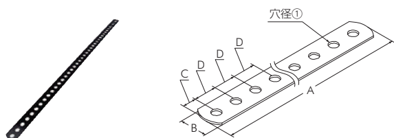
フリープレート ストレート 20X500
