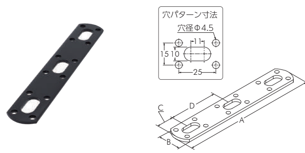
ジョイントプレート B-8
