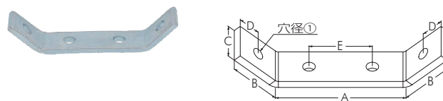
ミニチュア 火打ち 30・40・55mm
