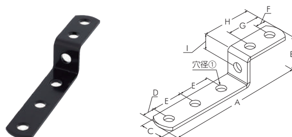
ジョイントプレート F-3
