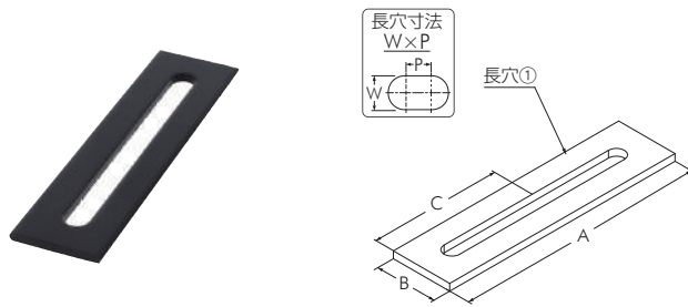
ジョイントプレート G-2
