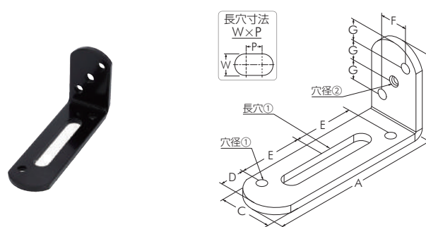
ジョイントプレート J-4
