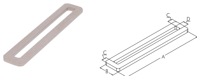
フリーポイント金具 プレート 小・大
