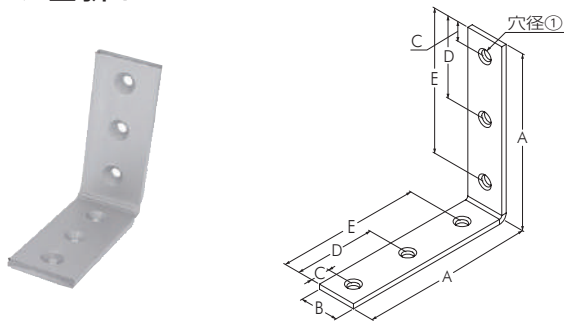
アルミ 金折れ 75mm
