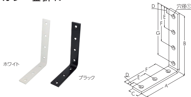
カラー金折れ
