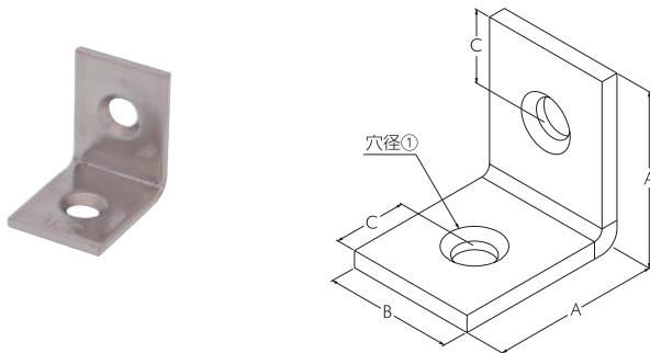
ステン 金折れ 20 x 20mm
