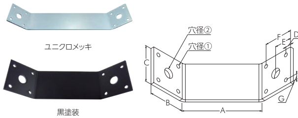
火打ち金具
