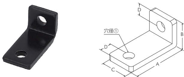
ミニジョイント アングル K-12
