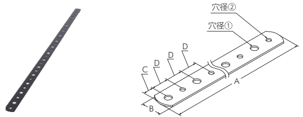
フリープレート チドリ 15X400
