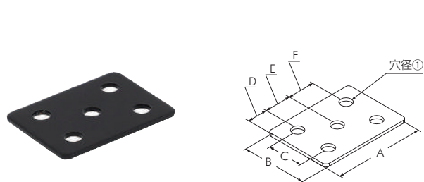
ミニジョイント 平板 M-1
