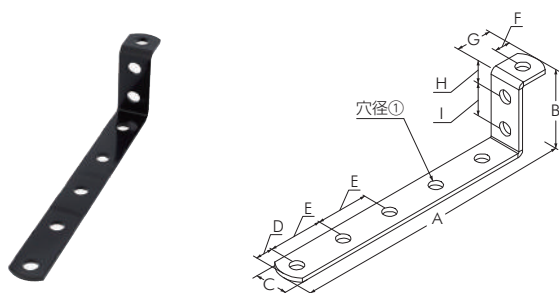
ジョイントプレート F-4
