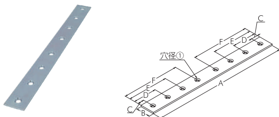
ユニクロプレート 240・300 mm
