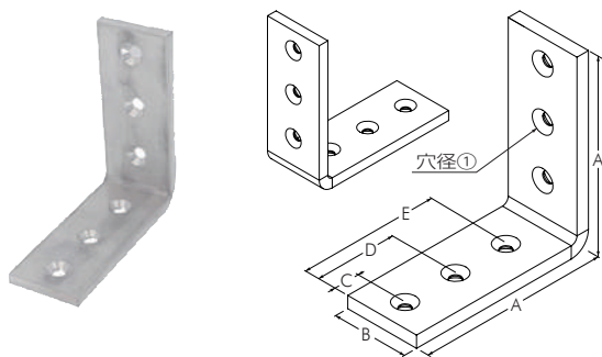
アルミ 両皿 金折れ 75mm
