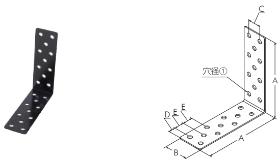
ミニジョイント 金折れ N-3
