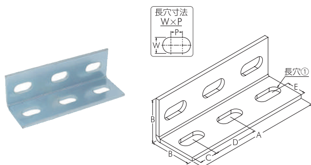
ユニクロ ファンブル 90mm
