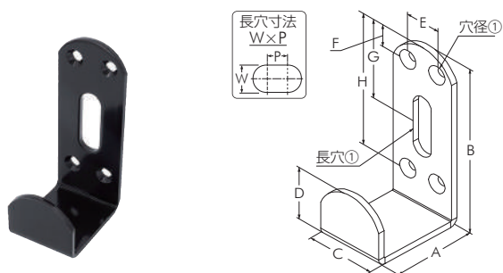
ジョイントプレート C-5
