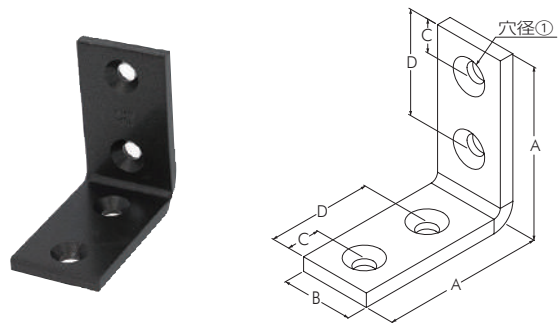
アルミ 金折れ ブラック 45・60・75mm
