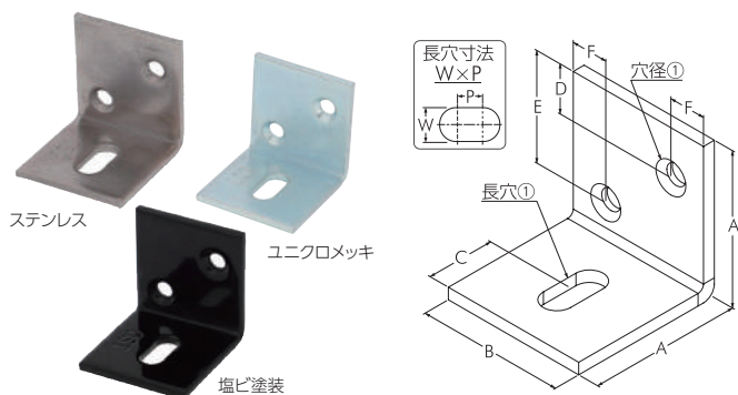
金折れ鋼板 縦穴
