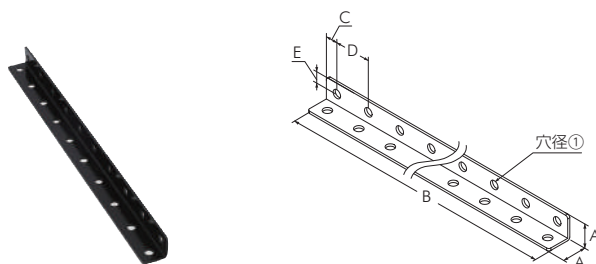
ミニジョイント アングル L-6
