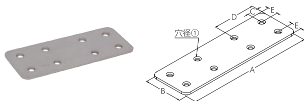
ステン 幅広プレート 90・120mm
