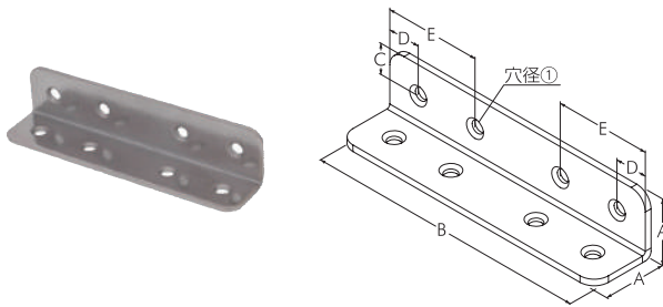
ステン アングル 90・120・150mm
