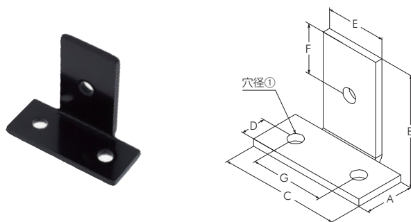
ジョイントプレート E-3
