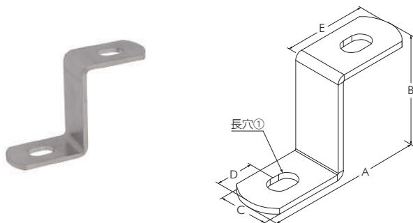
ジョイントプレート H-3
