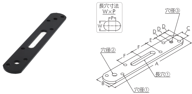
ジョイントプレート J-7
