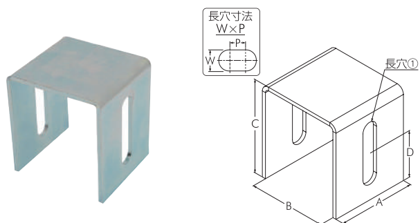
ユニクロ ルーズ金具
