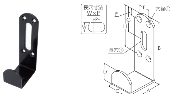
ジョイントプレート C-6
