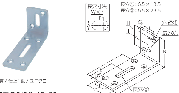
幅広万能金折れ 40x80mm
