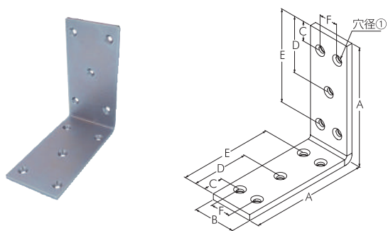
ユニクロ 幅広金折れ 120～180mm
