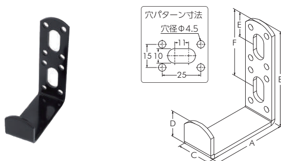
ジョイントプレート C-3
