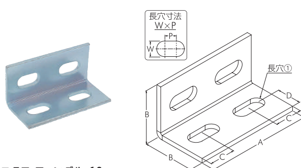
ユニクロ ファンブル 60mm
