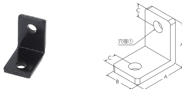
ミニジョイント アングル K-11
