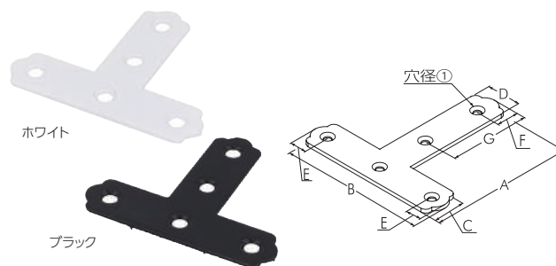
カラーT字 小・中・大
