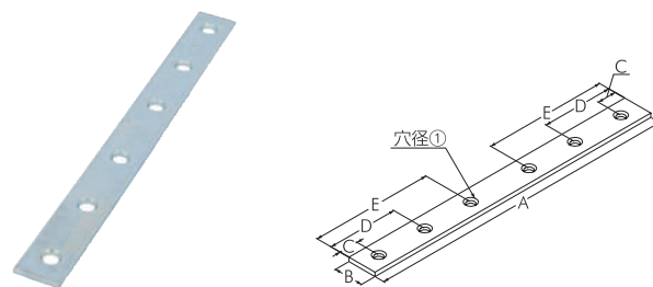
ユニクロプレート 180 mm
