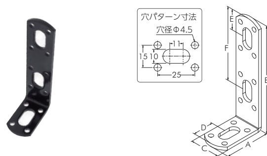
ジョイントプレート B-4
