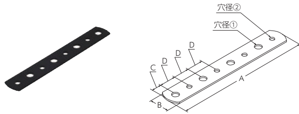
フリープレート チドリ 15X100
