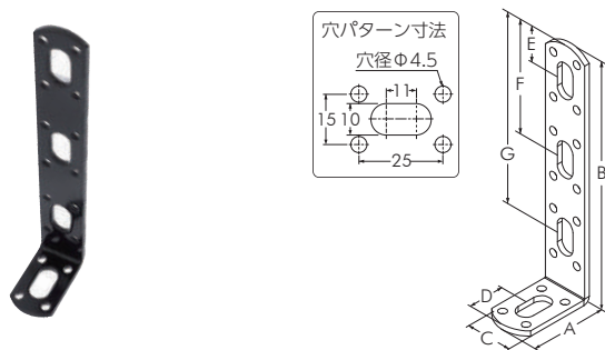
ジョイントプレート B-5
