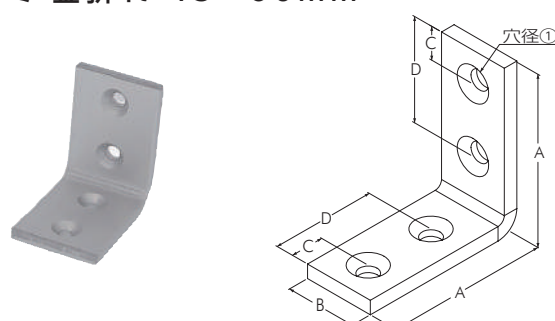
アルミ 金折れ 45・60mm
