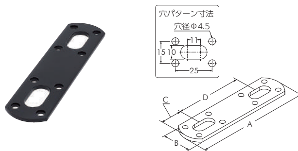
ジョイントプレート B-9
