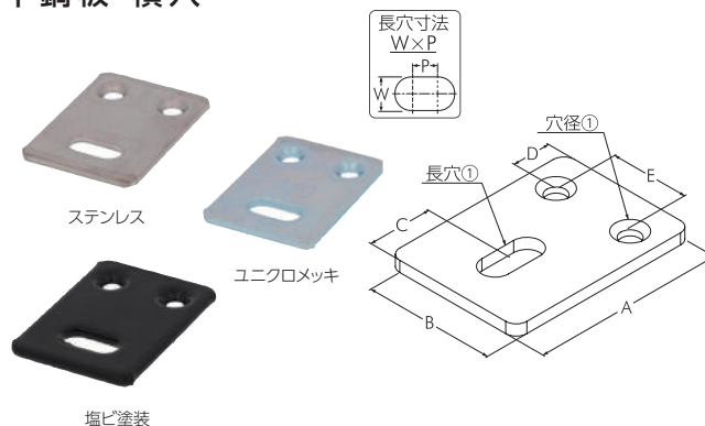
平鋼板 横穴
