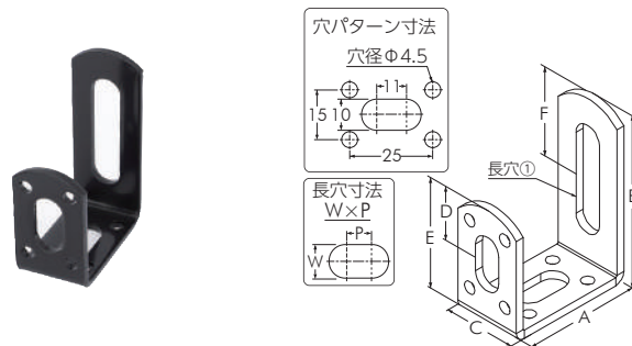
ジョイントプレート C-2
