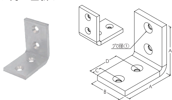
アルミ 両皿金折れ 45・60mm
