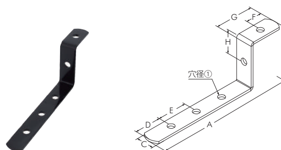
ジョイントプレート F-1
