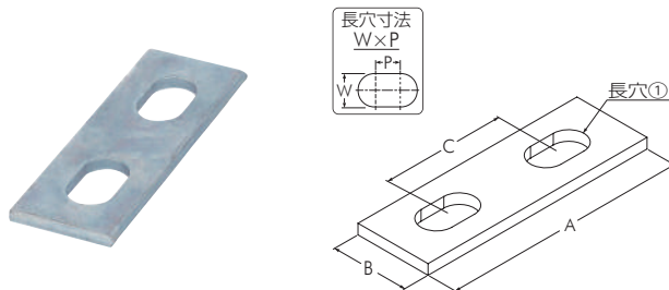
ユニクロ UB プレート
