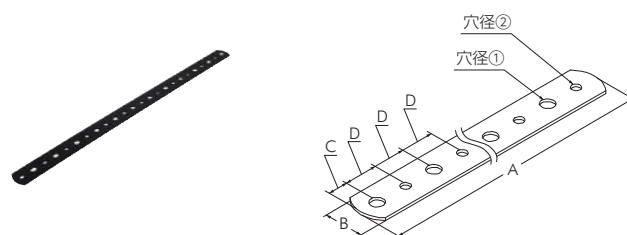
フリースプレート チドリ 20X300
